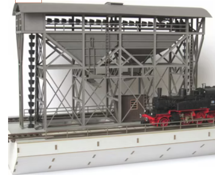
Art.-Nr. H10301: Hunt'sche Großbekohlungsanlage Bauart Antwerpen
